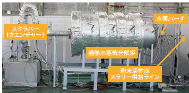
水素燃焼式高温過熱水蒸気分解処理試験装置
