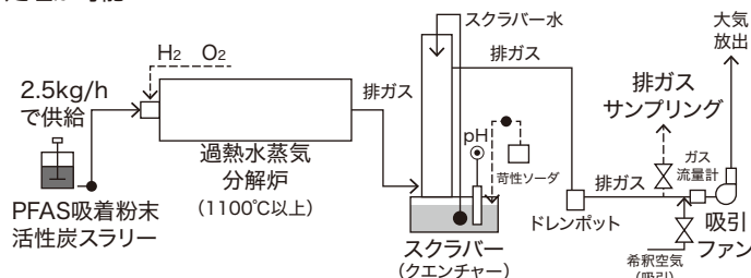
図 高温過熱水蒸気分解処理試験装置概要
