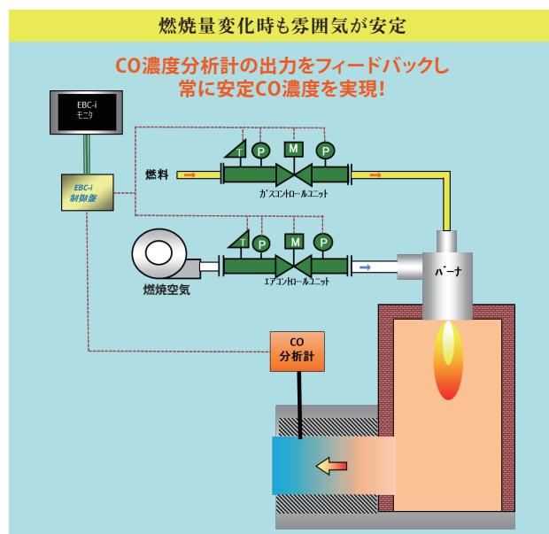
図1. DXガス発生装置におけるEBC-i制御装置の使用例
