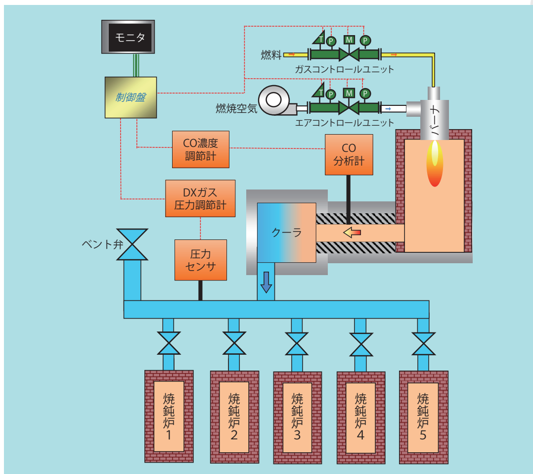
図3. 多数の焼鈍炉向けDXガス発生装置における、EBC-i制御装置の使用例
