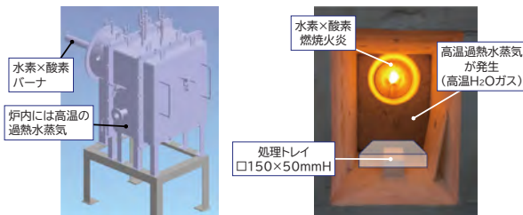
〈試験装置正面〉
