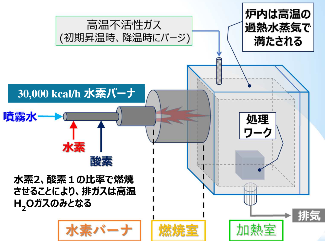
図1.過熱水蒸気試験装置正面図および概略図
