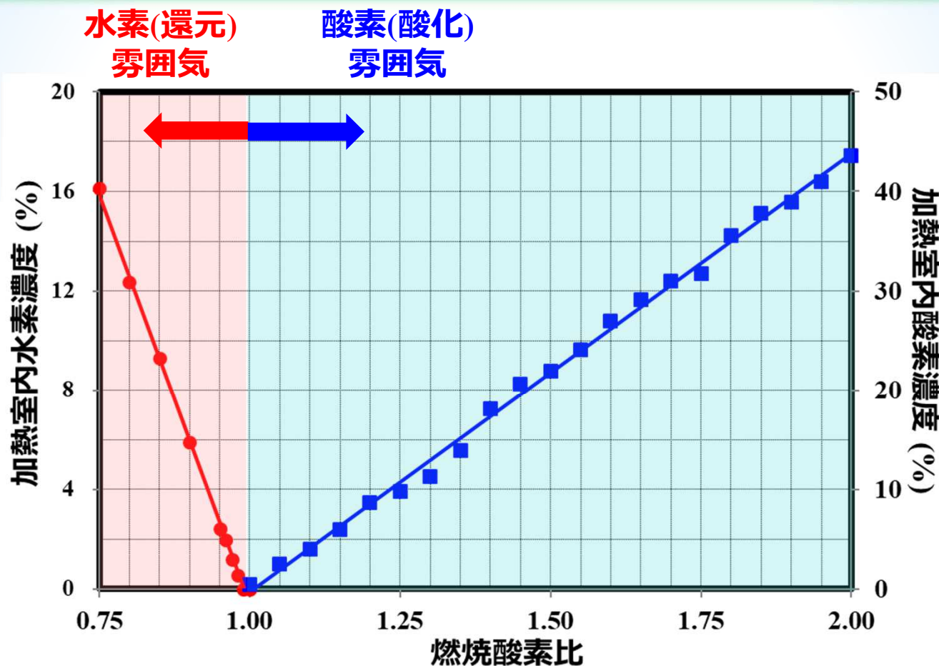
グラフ3. 燃烧酸素比の変化による加熱室内水素・酸素濃度
