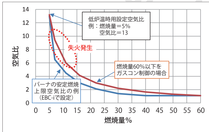
図3. 高過剰空気設定例
