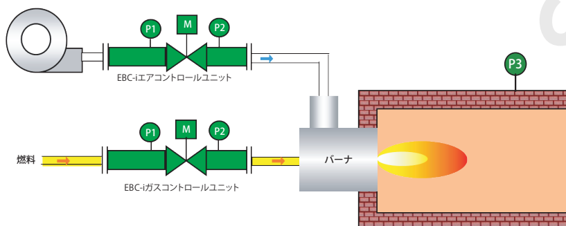
図7. 燃焼室にP3圧力センサーを取り付けた例
