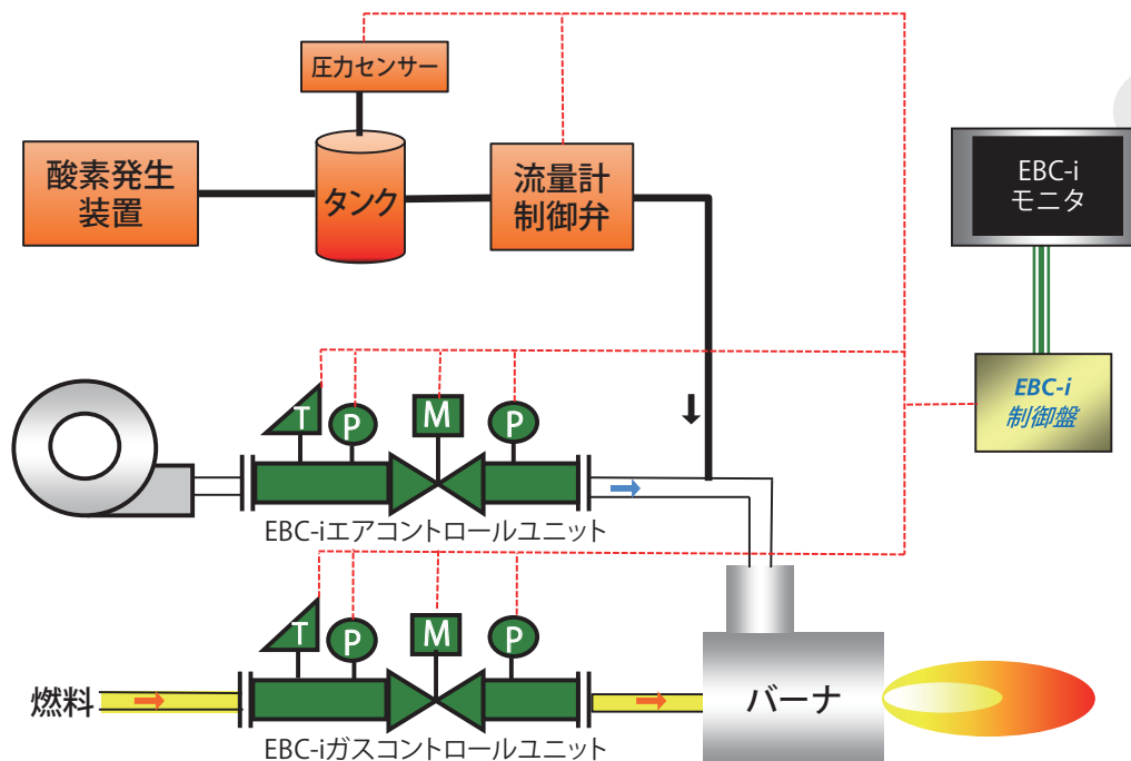
図6. 酸素富化燃焼への適用例
