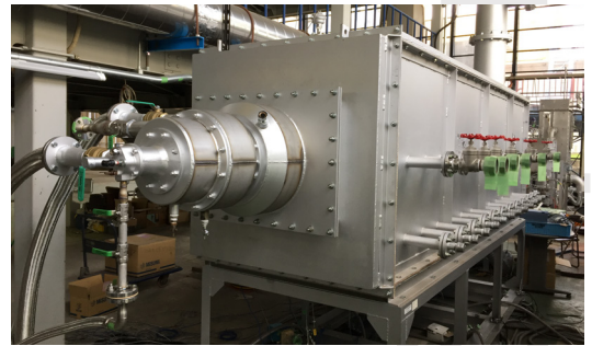
実験用バーナ
